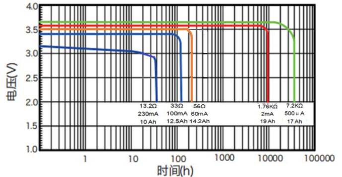
2. 在不同放电电流、温度条件下的电压曲线图 (在放电的稳定阶段)
