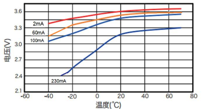
3. 在不同温度和电流条件下的容量曲线图 (截止电压为 2.0V)
