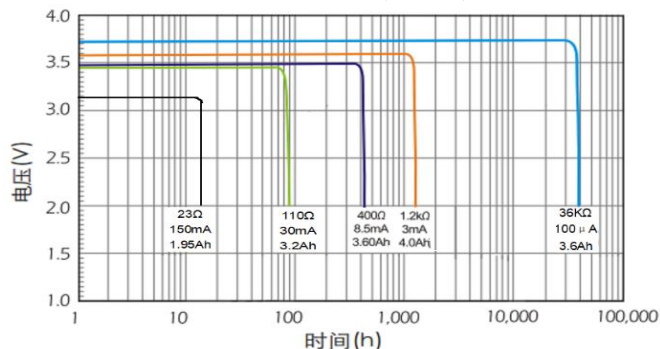
1. 在+25℃下典型放电曲线 (中间值)
