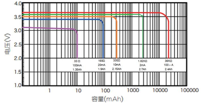
1. 在+25℃下典型放电曲线 (中间值)
