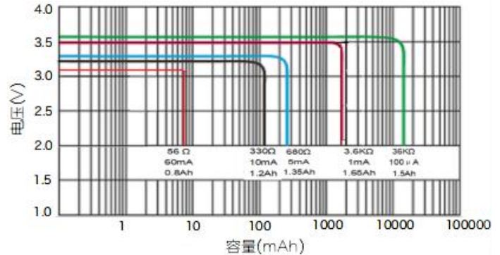
1. 在+25°C下典型放电曲线 (中间值)
