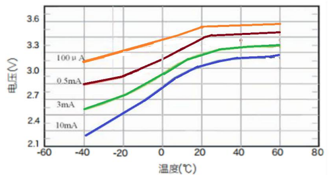
3. 在不同温度和电流条件下的容量曲线图 (截止电压为 2.0V)
