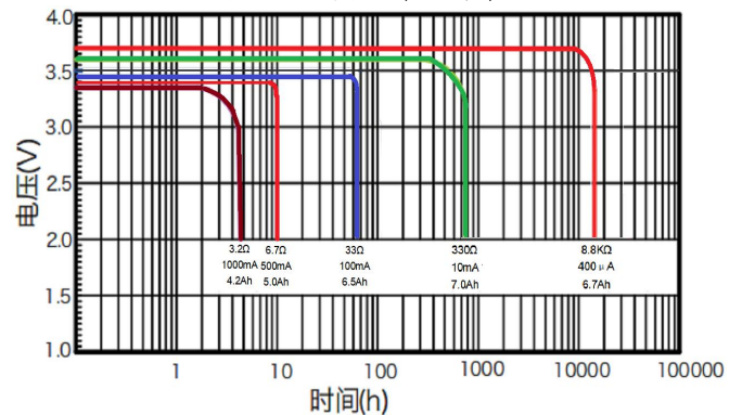
2. 在不同放电电流、温度条件下的电压曲线图 (在放电的稳定阶段)
