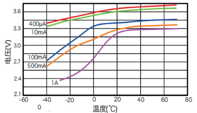
3. 在不同温度和电流条件下的容量曲线图 (截止电压为 2.0V)
