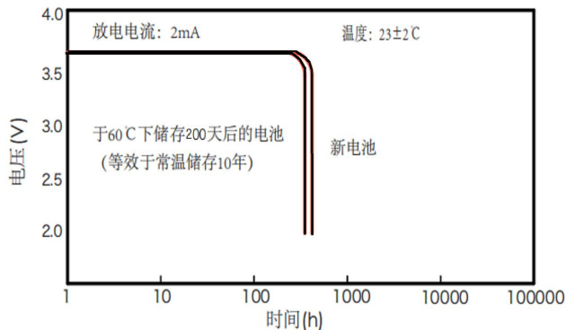
4. 贮存特性
