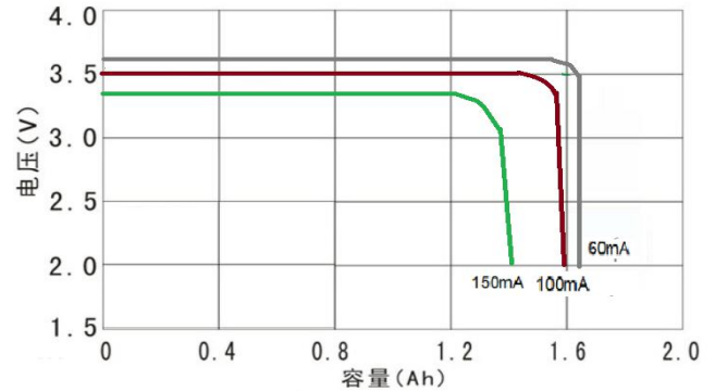
1. 在+135℃下典型放电曲线 (中间值)
