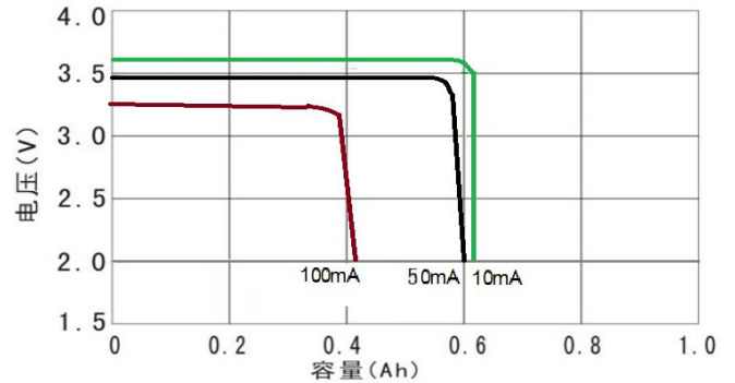
1. 在+135℃下典型放电曲线 (中间值)
