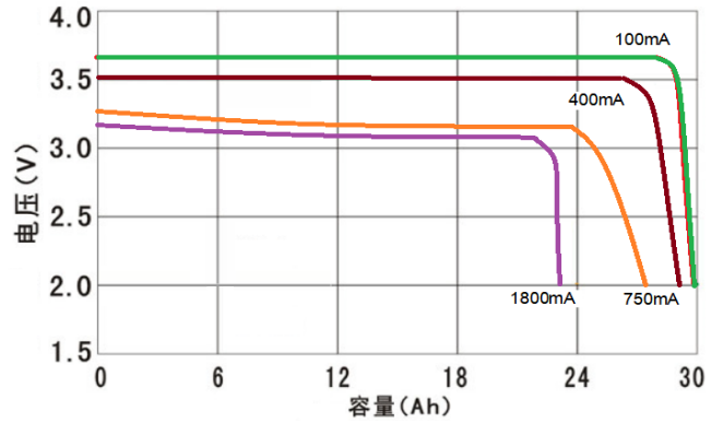
1. 在+135°C下典型放电曲线 (中间值)
