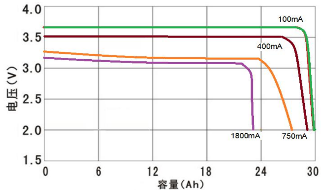
1. 在+135℃下典型放电曲线 (中间值)
